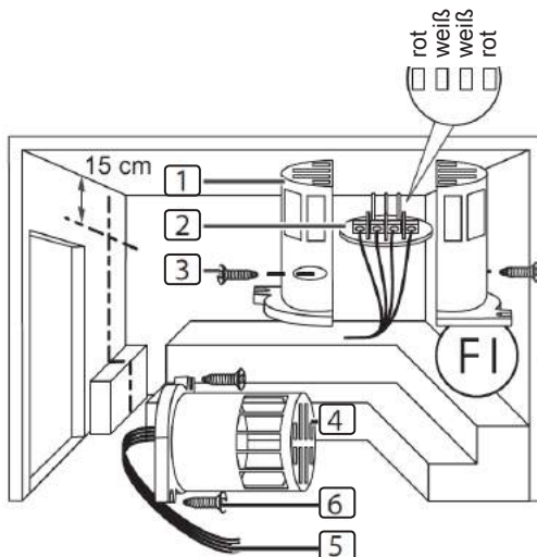
Abb.8 Montage des Ofenfühlers
