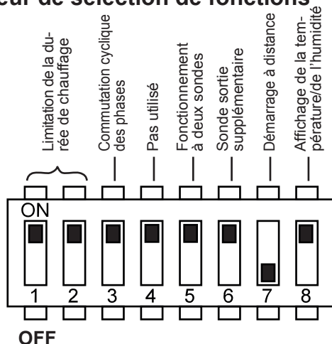
Fig. 11 Commutateur de sélection de fonctions - réglage standard
