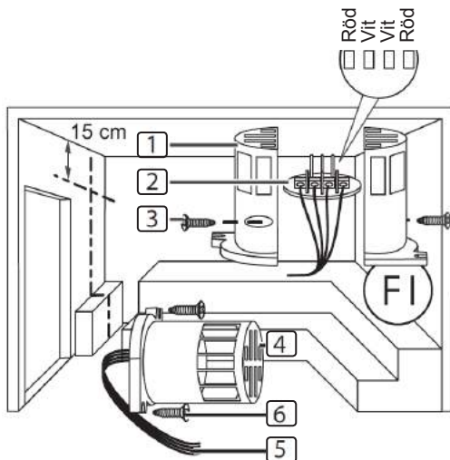
Bild 8 Montera aggregatgivare
