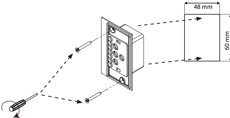
Kuva 6 Hallintalaitteen lisälähdön asennus (valinnainen)
