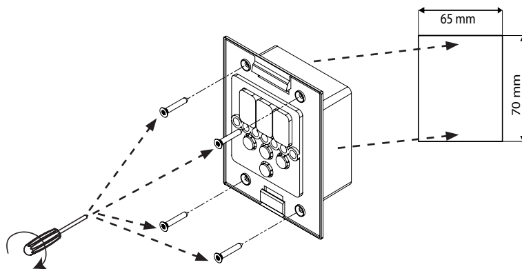
Fig. 5 Montaggio dell'unità di comando Pro D
