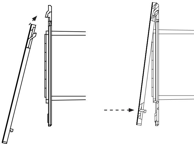
Abb.7 Montage Bedienteil
