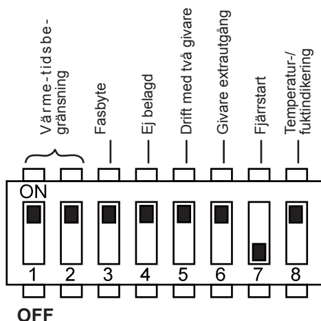
Bild 11 Funktionsomkopplare - standardinställning
