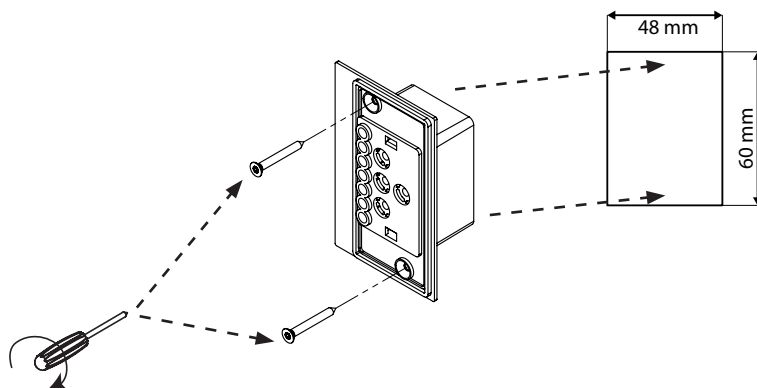
Fig. 6 Montaggio dell'uscita supplementare dell'unità di comando (opzionale)
