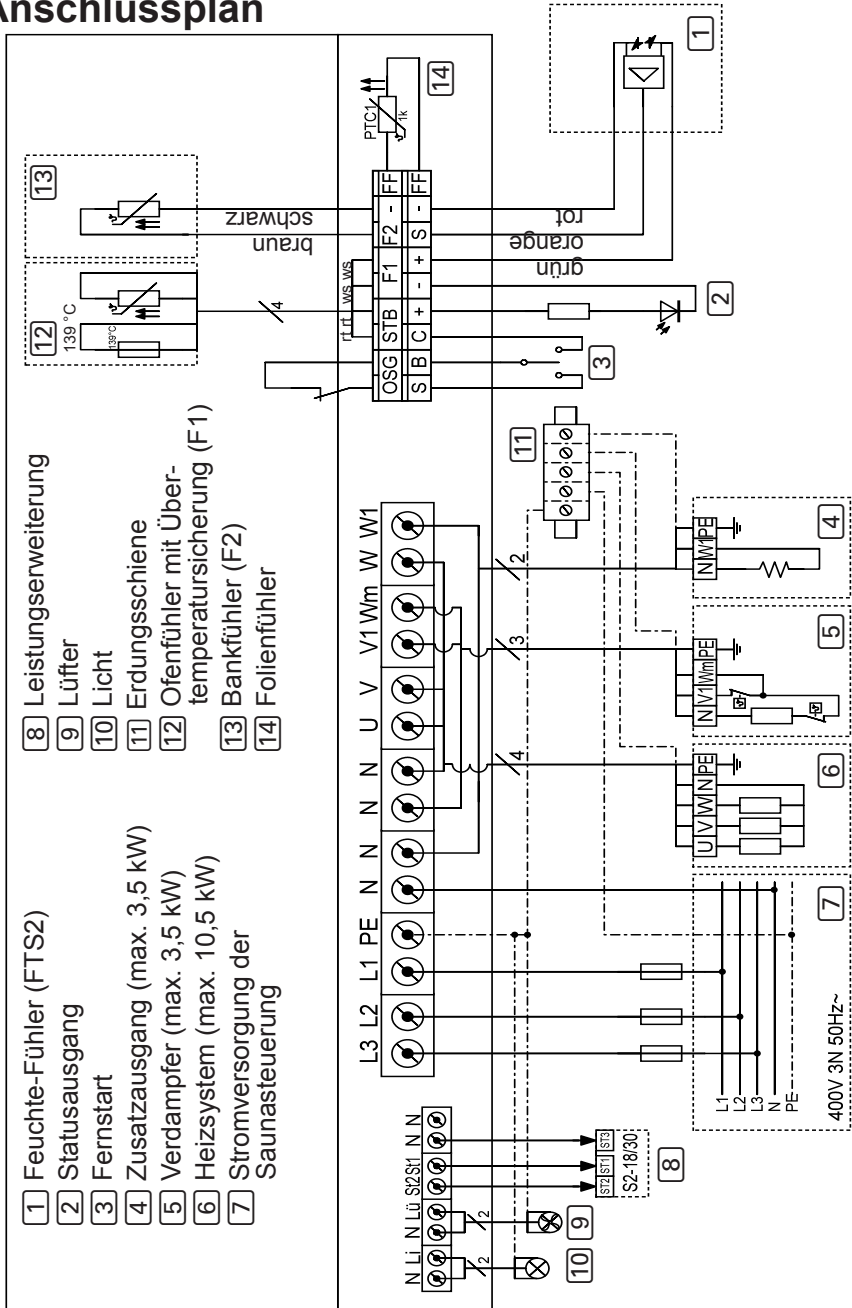
Abb. 10 Anschlussplan
