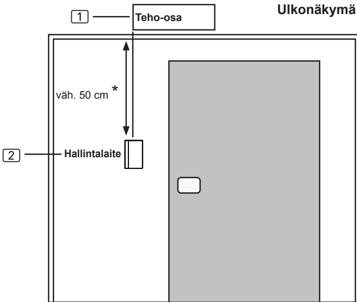
Kuva 4 Hallintalaitteen paikka
