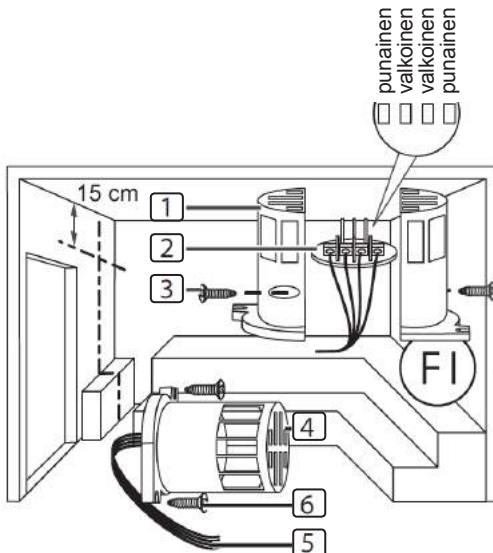
Kuva 8 Kiuasanturin asentaminen
