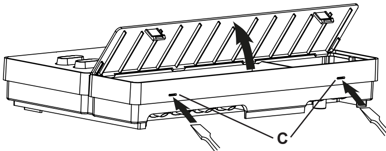
afb. 3 Behuizingsdeksel verwijderen
