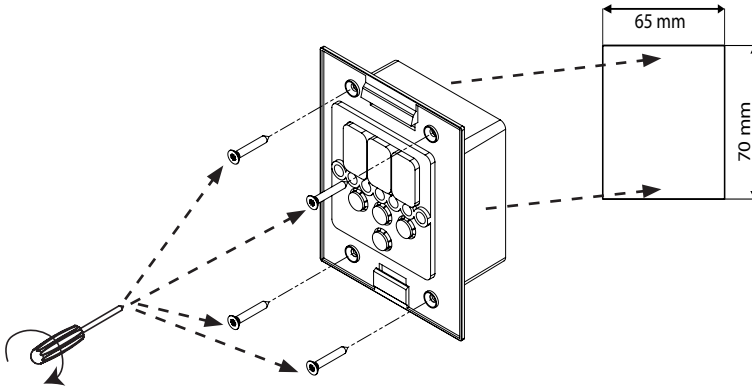
Bild 5 Montering av manöverenhet Pro D
