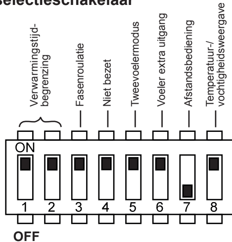
afb. 11 Functieschakelaar - standaardinstelling
