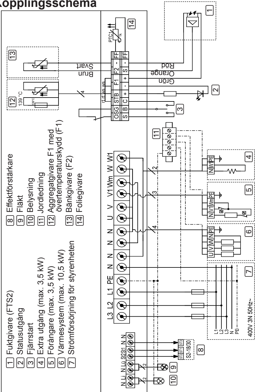
Bild 10 Elschema
